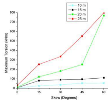
Fig 7: Maximum Torsion Class70RW+A
